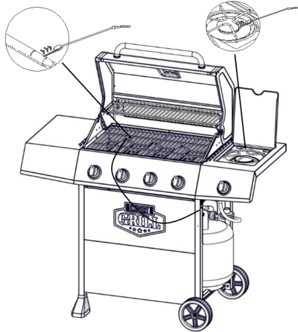
Quemador Principal
