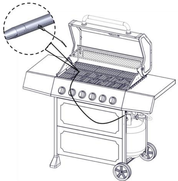
Quemador principal
