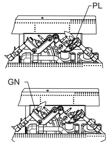
Fig. 26 - Piloto
