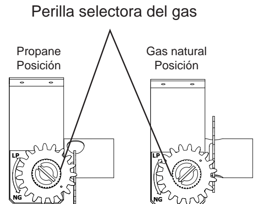
Fig. 13 - Válvula selectora
