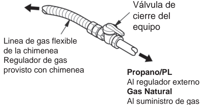
Fig. 16 - Instalación de la línea flexible de gas a la válvula de cierre del equipo
